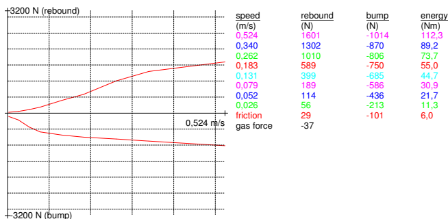
График характеристик передних амортизаторов
